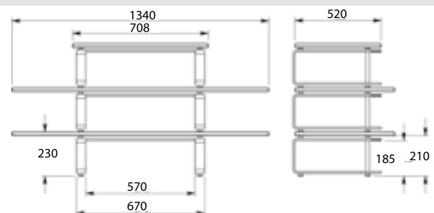
ГАБАРИТНЫЕ РАЗМЕРЫ в мм
