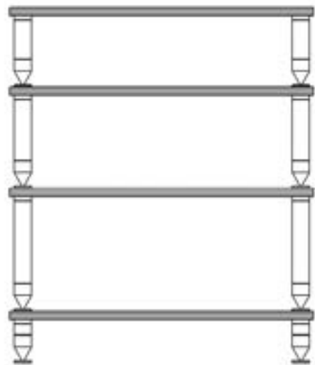
Base 120 + Modul 270 + Modul 220 + Modul 170
