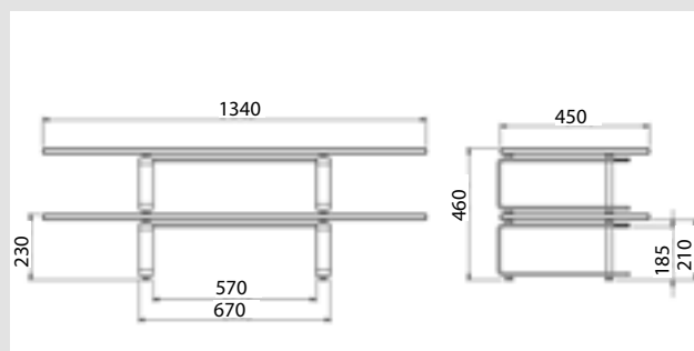
ГАБАРИТНЫЕ РАЗМЕРЫ в мм
